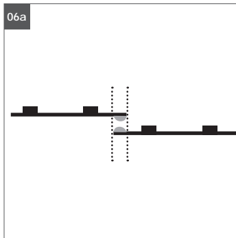
06a. Verbindung von Teilmodulen durch Auflöten einer Brücke. An den Lötstellen oben (Bild 06b) und unten (Bild 06c) miteinander verlöten. Lötstellen unten werden erst sichtbar wenn man die Schutzfolie abzieht. Bitte Schutzfolie nicht komplett abziehen , damit das FLEXY nicht die Klebkraft verliert! Achtung: Es dürfen an eine Einspeisung maximal 5m Flexmodul gehängt werden, danach muss neu eingespeist werden. 06a. Segments can be connected by soldering of a bridge. Solder up the upper soldering point (pict. 06b) with the lower point (pict. 06c). Soldering points become visible as soon as protection foil is taken off. Don't take off the foil completely as not to lose the adhesive power of FLEXY. Attention! Maximum 5m of Flex strip can be installed with one feeder. For more, additional feeding is required.
