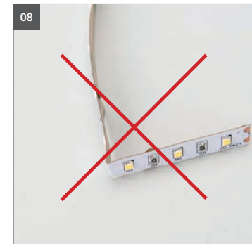
08. Nicht knicken, ein Knick zerstört die Leiterbahn. 08. Do not bend, bending will damage the conductors.
