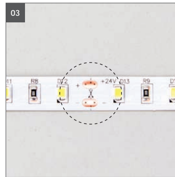
03. ... nur an bestimmten Stellen. 03. ... only at certain points.
